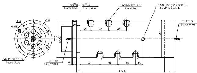
MAPH600S-02 尺寸图
