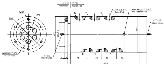
MAPH600S-03 尺寸图
