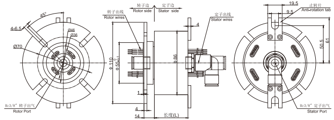
MAPH100-05 尺寸图
