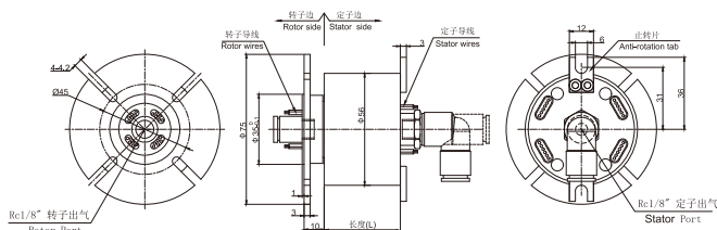
MAPH100-03 尺寸图
