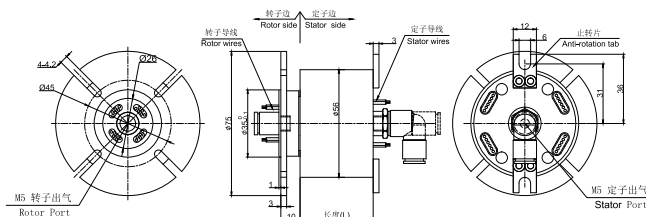
MAPH100-01 尺寸图
