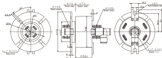
MAPH100-03 尺寸图
