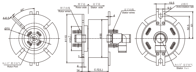
MAPH100-05 尺寸图
